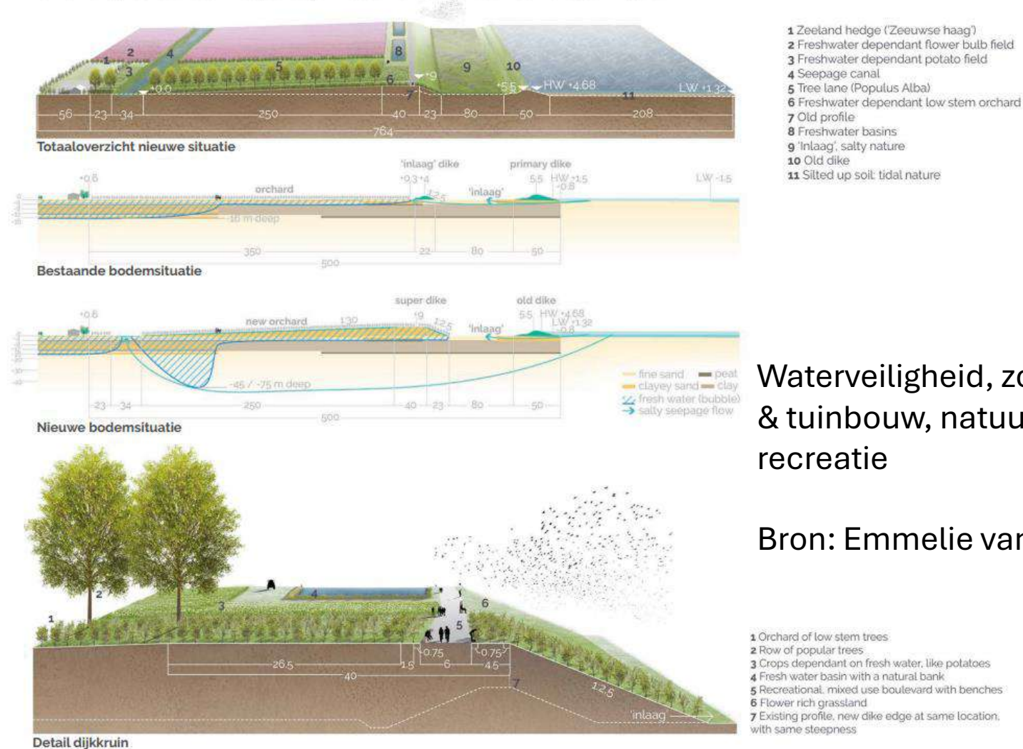
Ontwerp landbouw-superdijk : flauwe talud aan landbouwzijde
